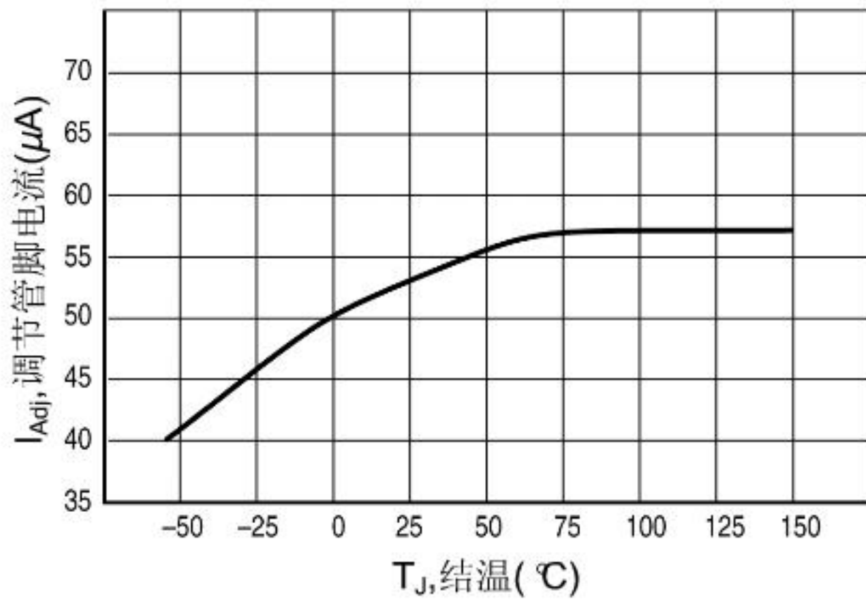
图 9. 温度稳定性
