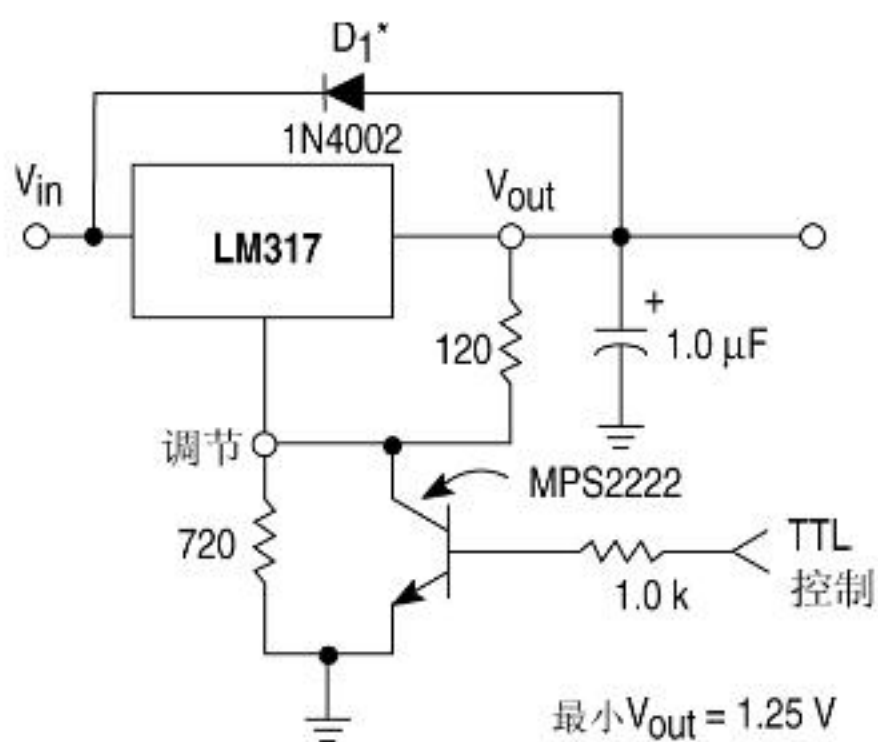
图 22. 5.0V 电子关断稳压器
