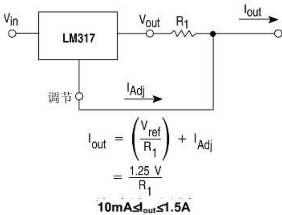
图 24.电流稳压器
