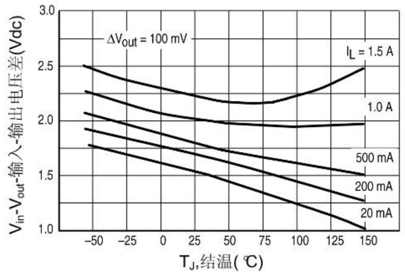
图 8. 压降电压
