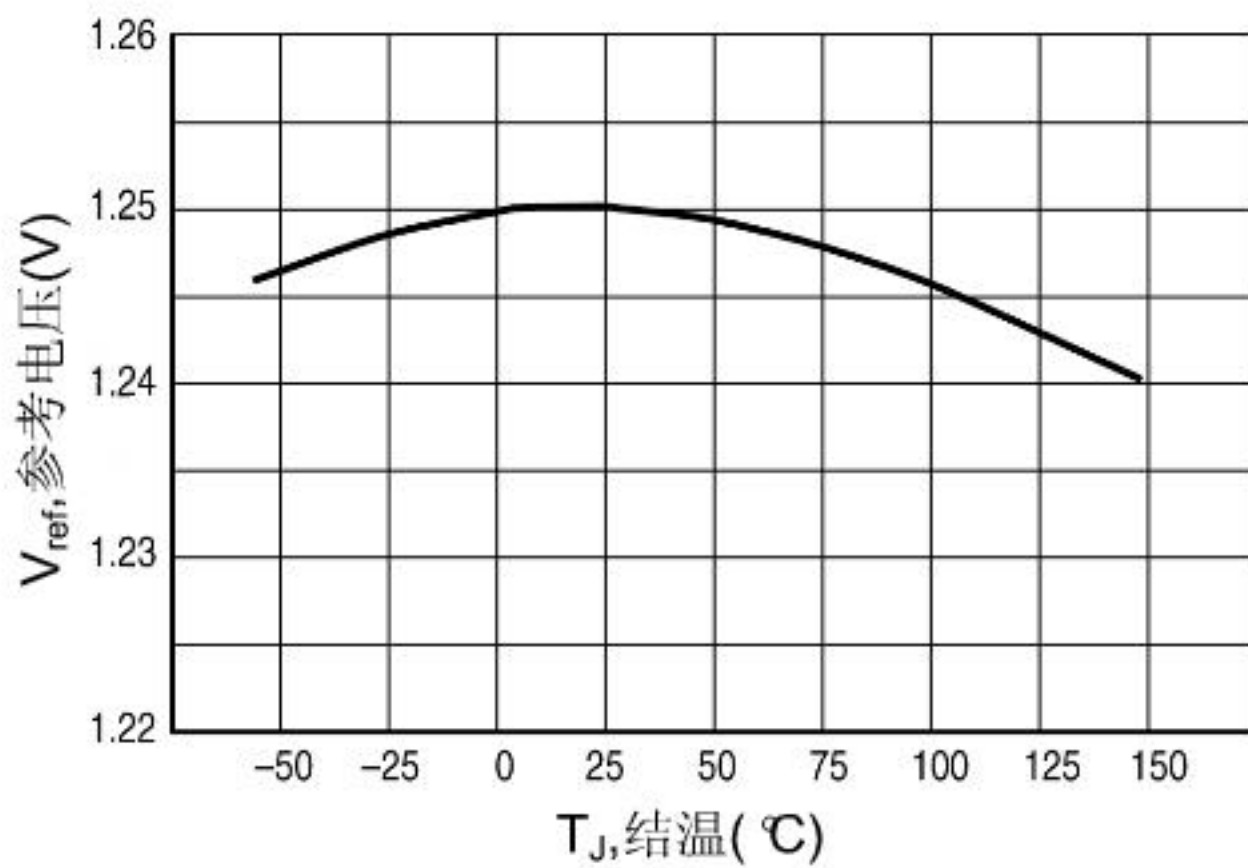
图 9. 温度稳定性
