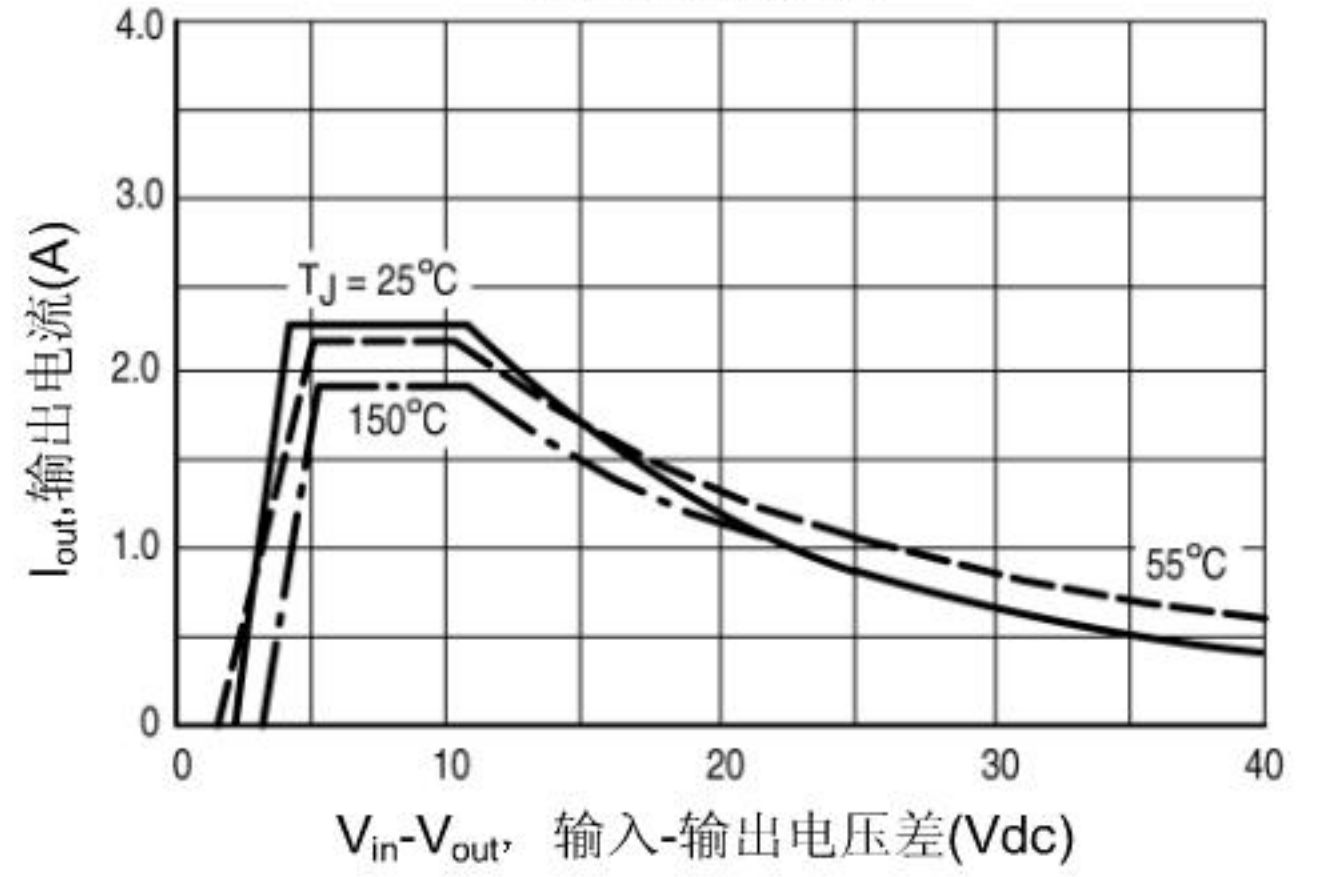
图 6. 电流限度
