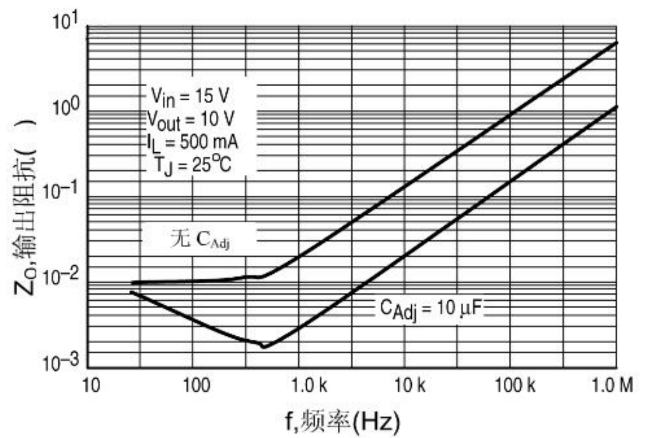
图 14. 输出阻抗
